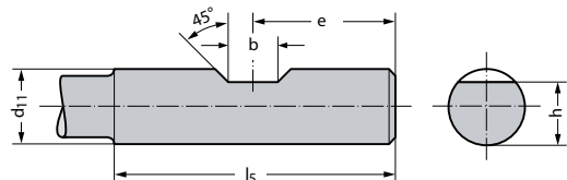
Форма HB для d 11 = 6–20 мм
