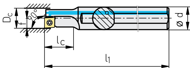
Схема правого инструмента
