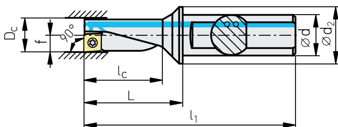
Схема правого инструмента
