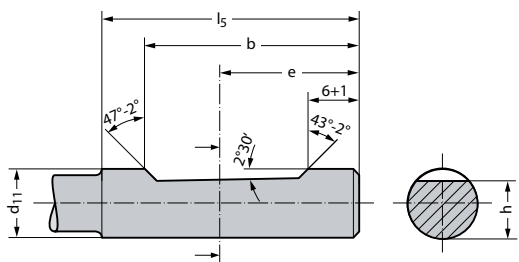
для d 11 = 25 мм
