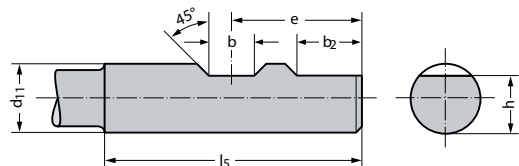
Форма HB для d 11 = 25 мм
