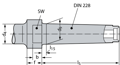
Базовый держатель МК DIN 2207
