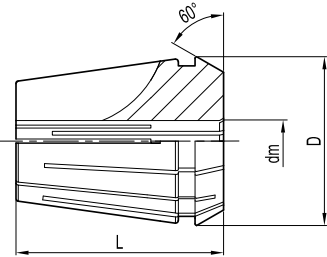
ER弹性筒夹 ER Collet
